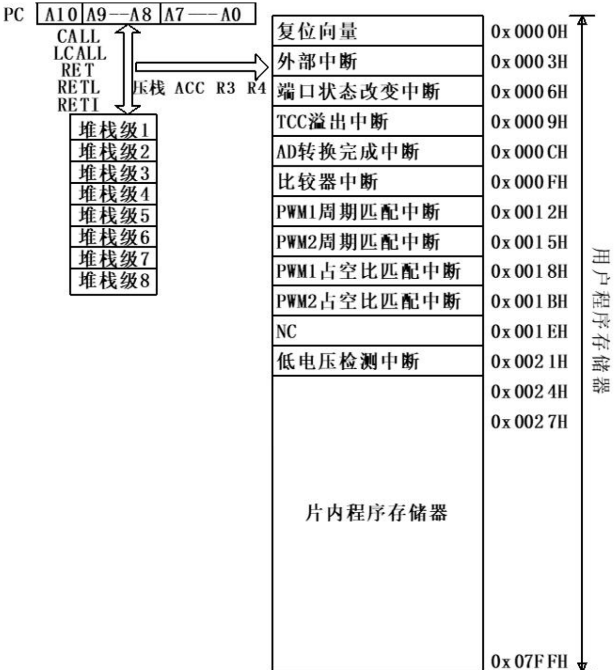
程序存储器区结构图
