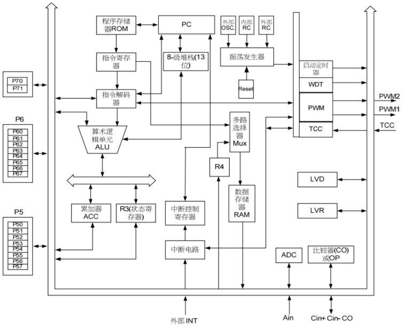
系统结构框图
